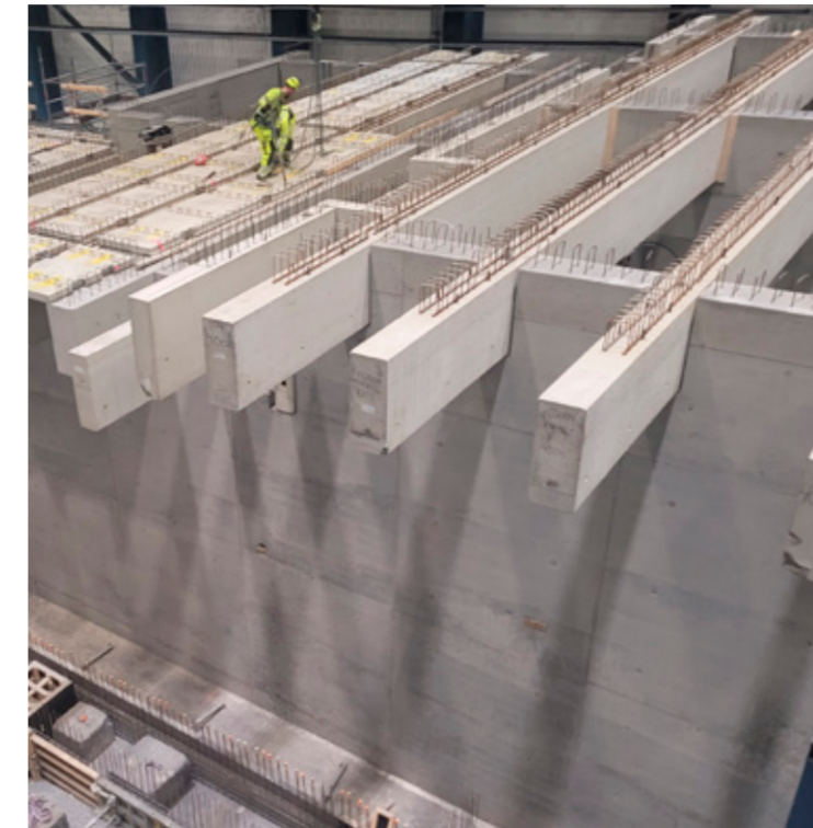
Montering av prefab till fundament.
